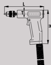
Typ PV (s hadicí)
